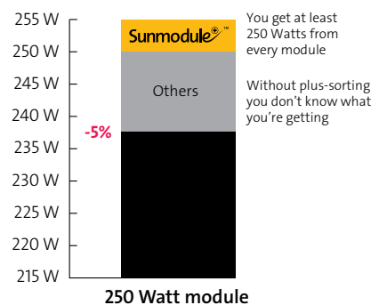
250 Watt module
